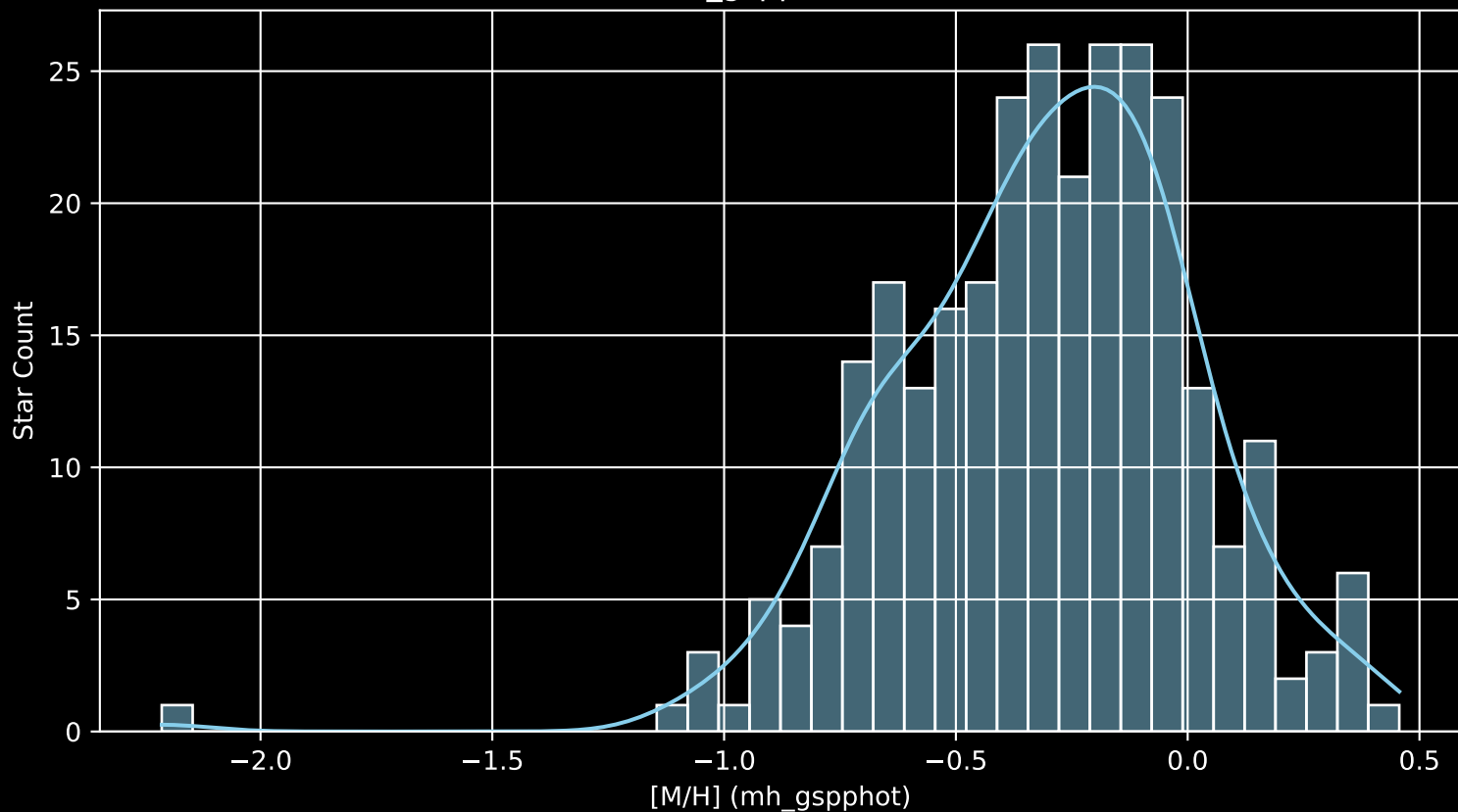
GALAH DR4 Field: [181] [M/H] (mh_gspphot) (n= 289)
