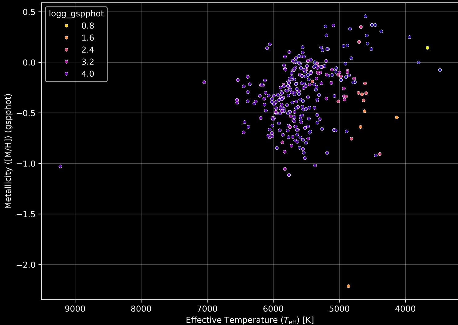
GALAH DR4 Field: [181] Stellar Population Parameters (n= 289)
